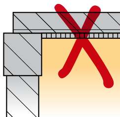
Vrijdragende betonvloer direct op zand
